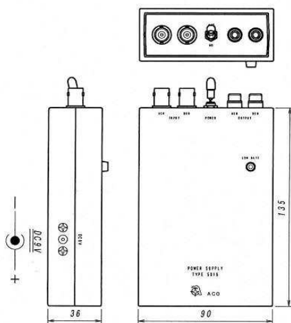
2CHマイクロホン電源 TYPE 5016 外観図
